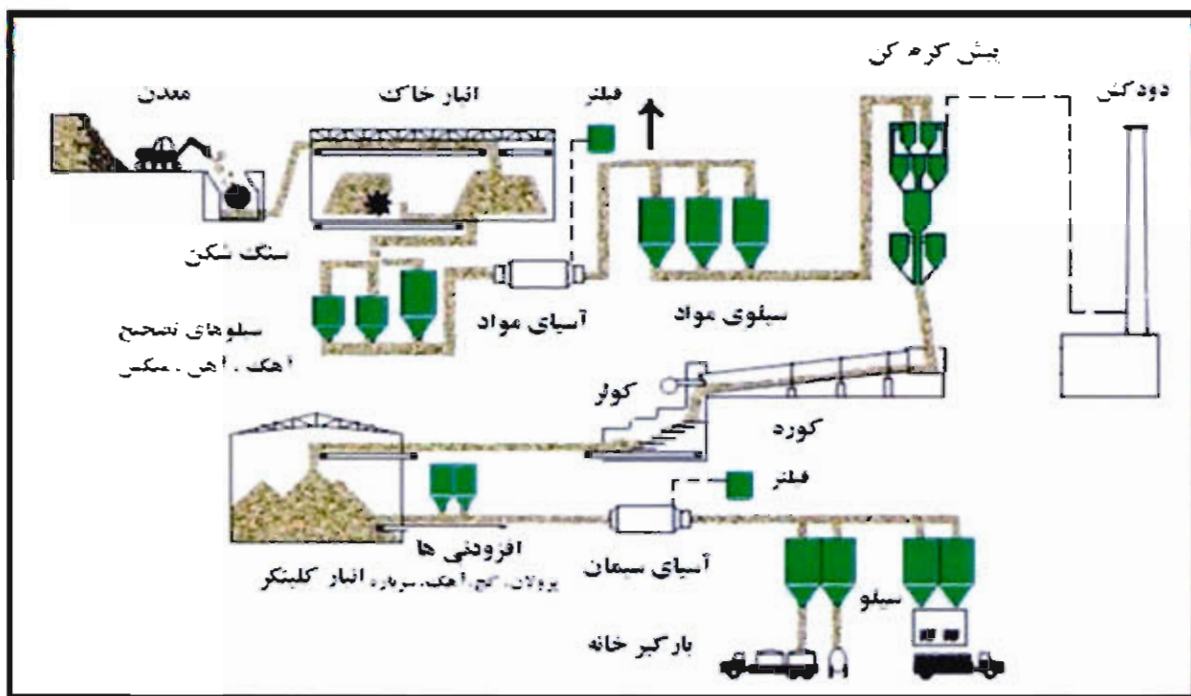
نمایه ۳۵- چرخه تولید سیمان
